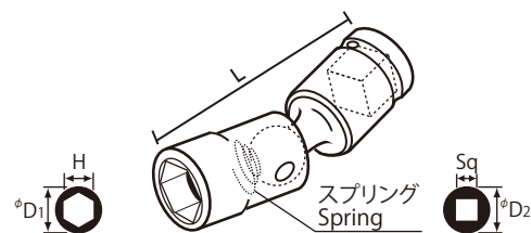
12.7Sq. ユニバーサルソケット Universal Sockets (Single Hex)
