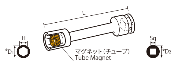
○ MT エクステンションタイプ Extension Sockets (Single Hex)
