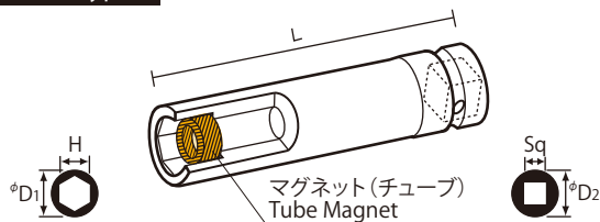
○ MT ディープタイプ Deep Sockets (Single Hex)
