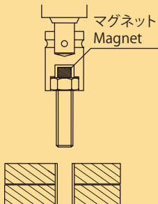
MP 圧入タイプ Fixed Type
