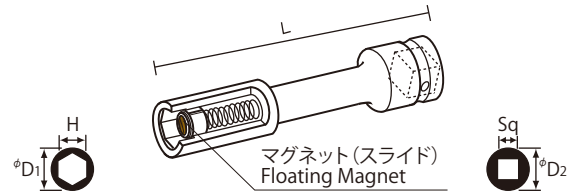
○ MS エクステンションタイプ Extension Sockets (Single Hex)
